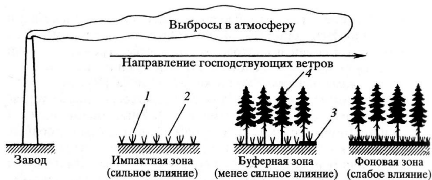
Рис. 2. Деградация лесных фитоценозов северной тайги под влиянием загрязнения атмосферы выбросами металлургического комбината: 1 – кустарнички; 2 – осыки; 3 – моховой покров; 4 – хвойные деревья (ель, сосна).
